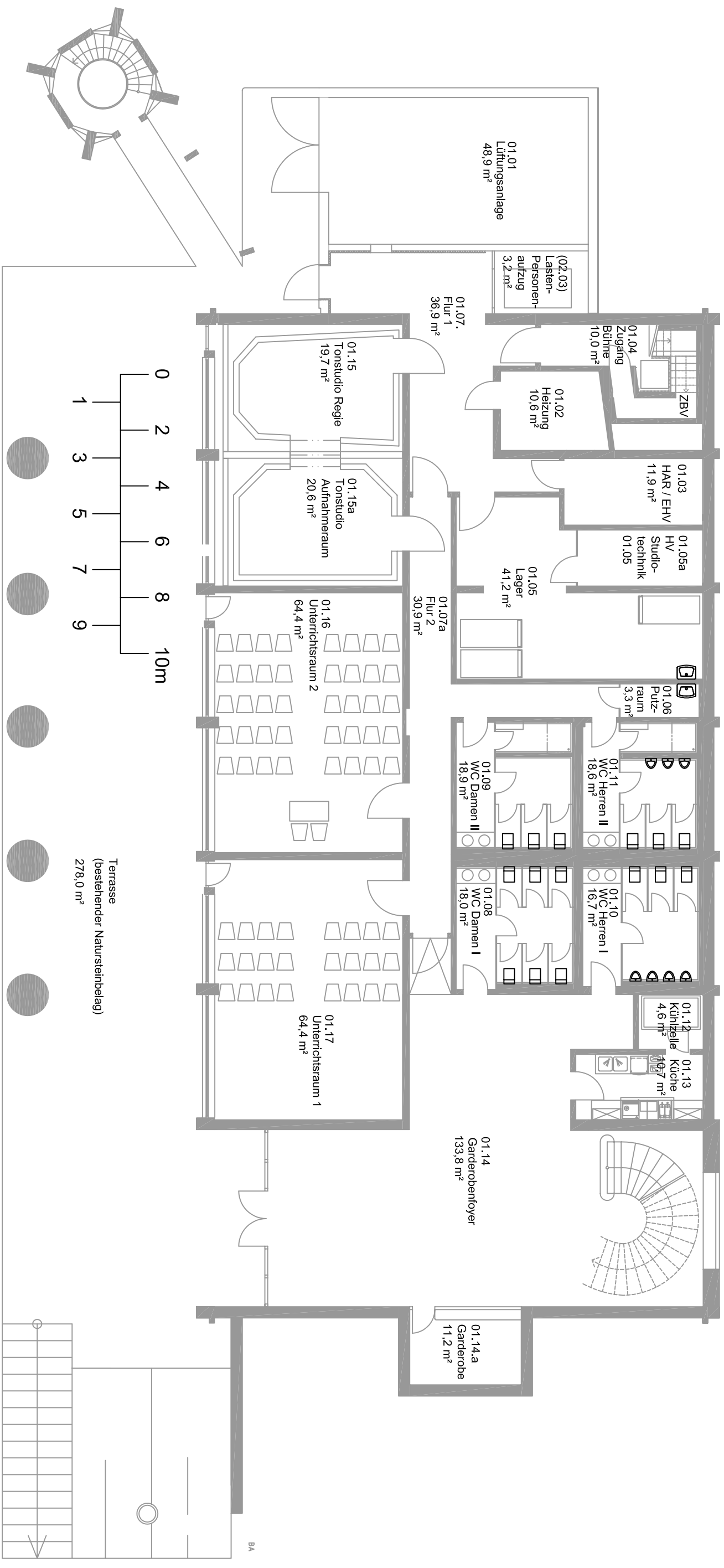
Akademiebühne Grundriss Gartengeschoß / UG M 1:150 (A3)
